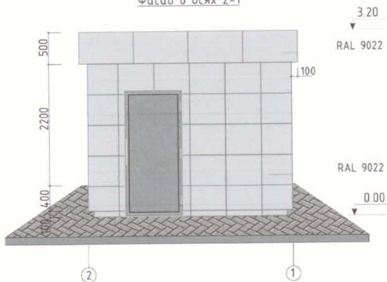
Фасад в осях 2-1
