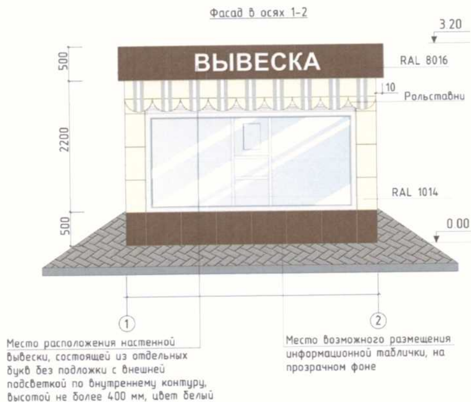
Паспорт отделки фасада:
