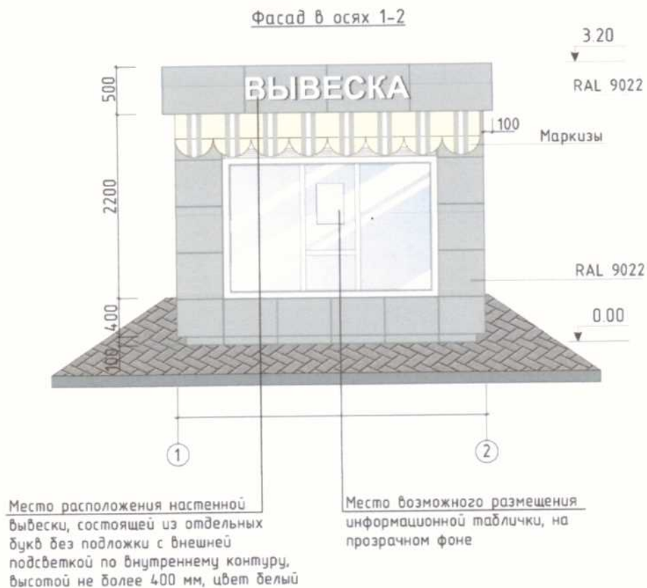
Паспорт отделки фасада:
